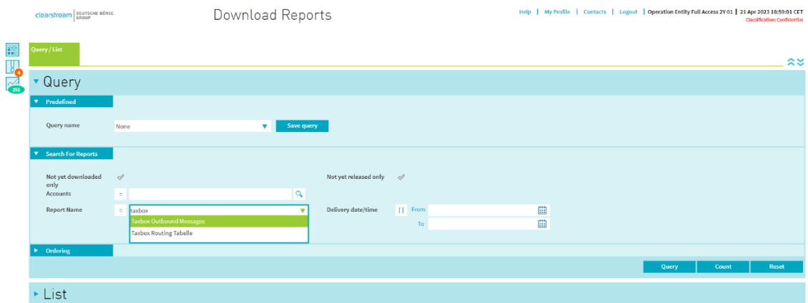
Abb. 4.3 Auswahlkriterien
