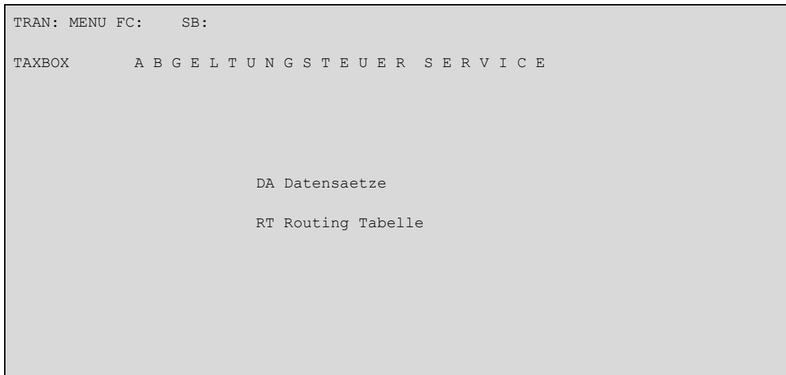
Abbildung 5.3: Taxbox Startmaske
